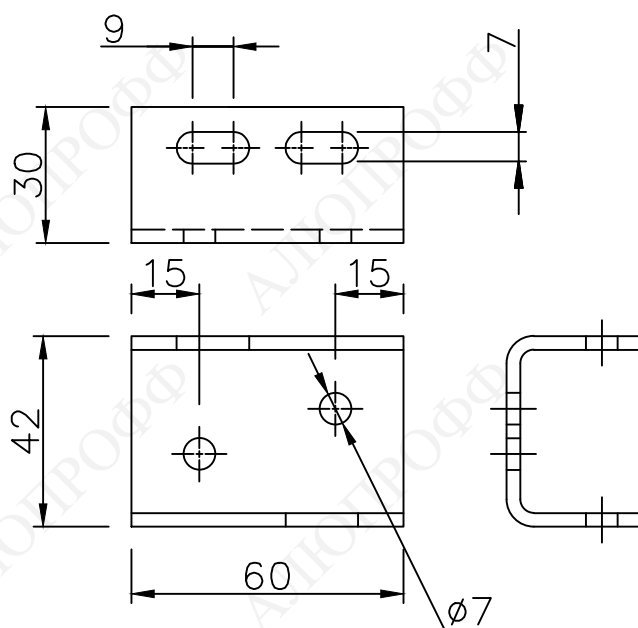
Кронштейн ALKU6030
