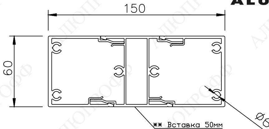
Ламель ALP60x150
