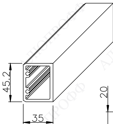
Ламель ALP35x45
