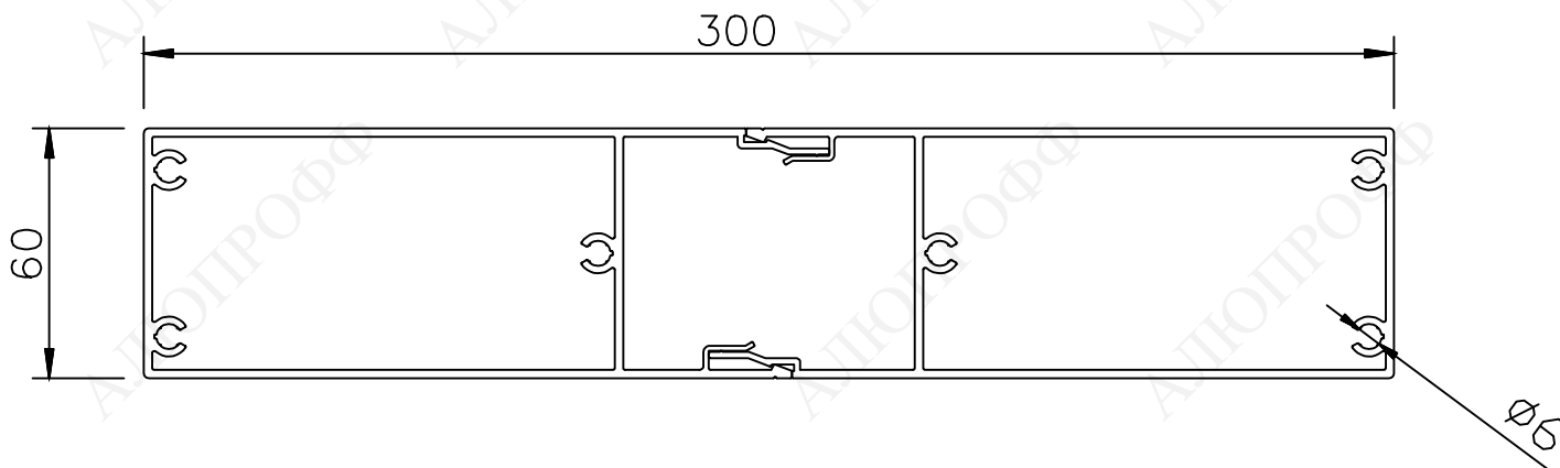
Ламель ALP60x300
