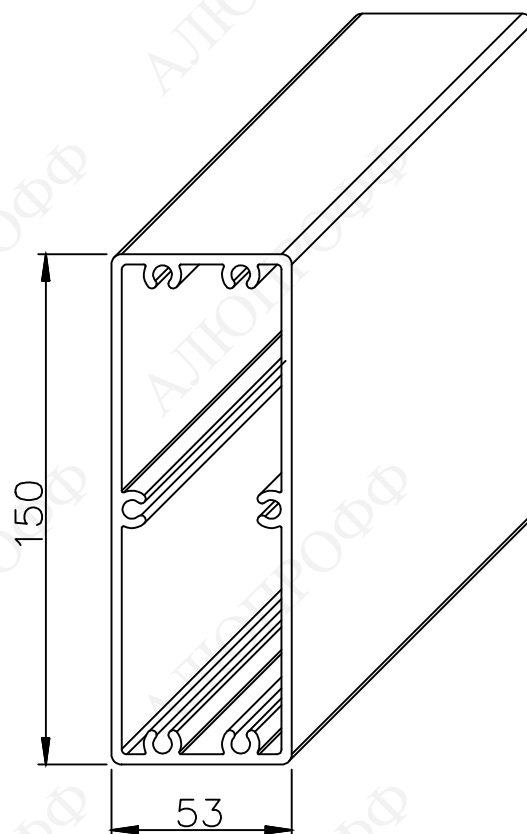
Ламель ALP53x150
