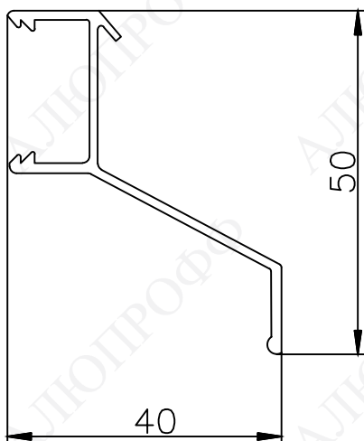
Ламель ALZ50x40
