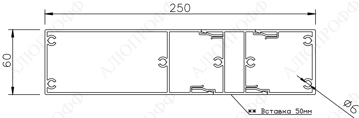
Ламель ALP60x250
