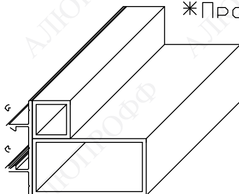
Ламель ALK50P *Проф.труба 20x20 *Проф.труба 60x30
