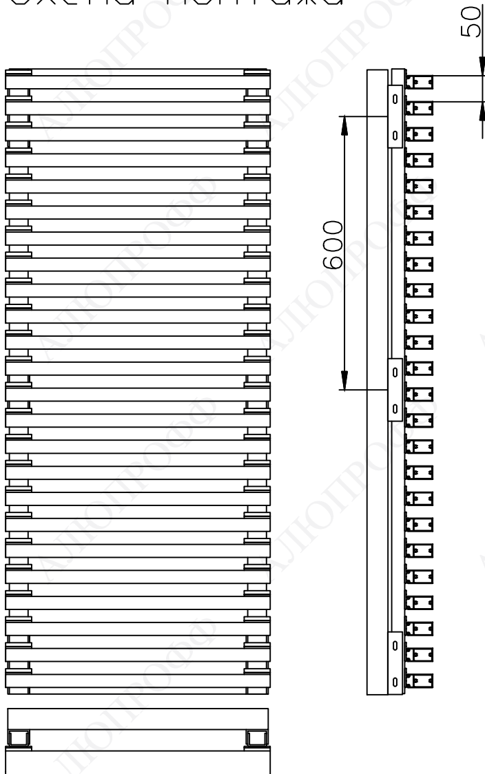
Схема монтажа
