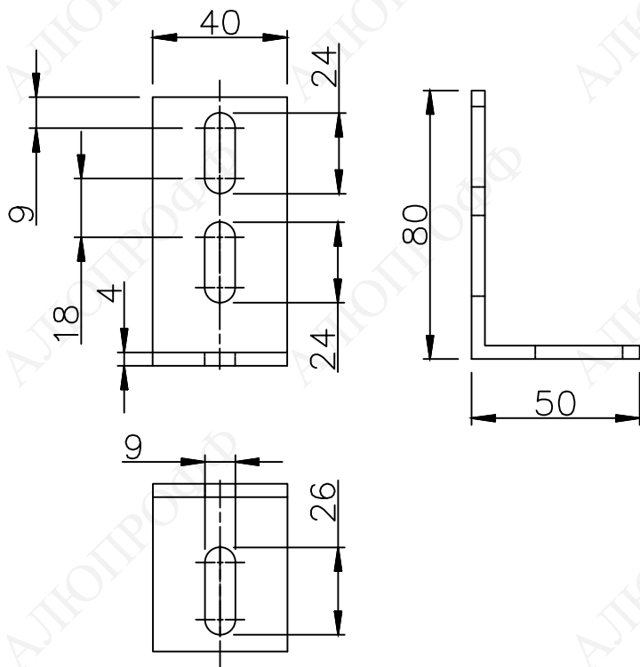
Кронштейн ALKL
