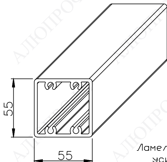
Ламель ALP55x55
