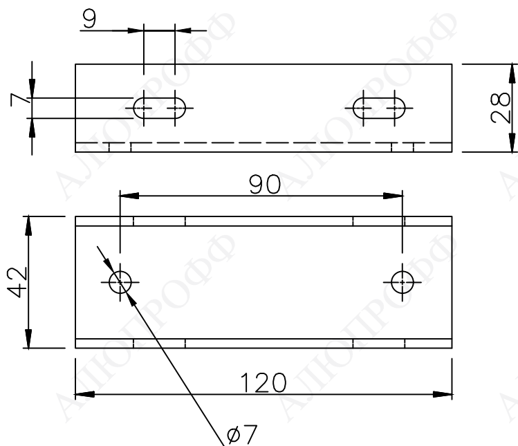
Кронштейн ALKU2842
