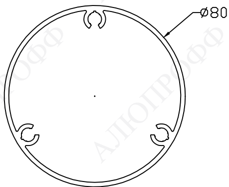
Ламель ALO 80
