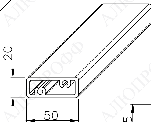
Ламель ALP20x50
