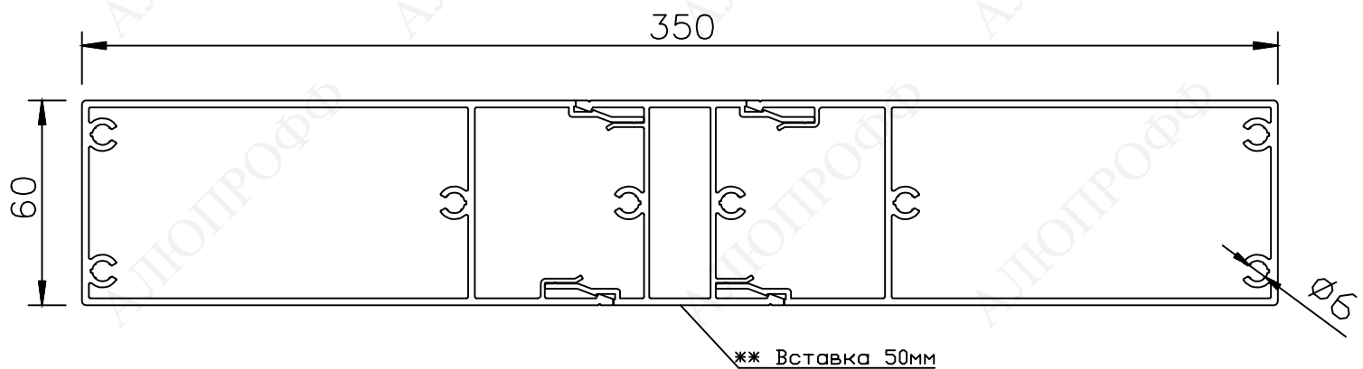
Ламель ALP60x350
